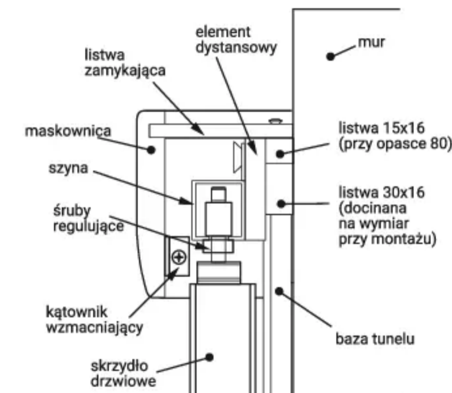
rys. 7 - Regulacja skrzydła przy pomocy śrub, zakończenie montażu
